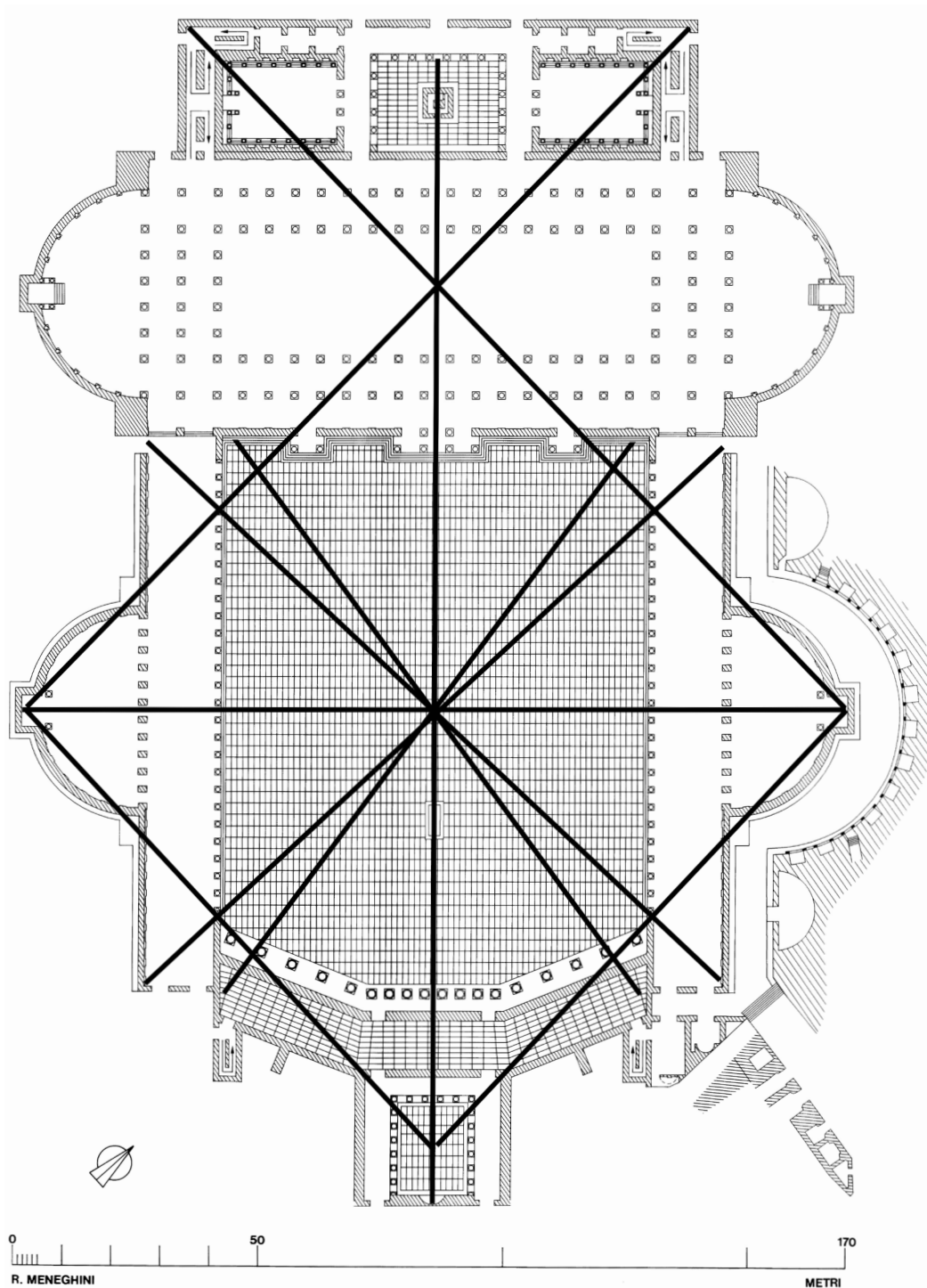
FIG. 28. Planimetria ricostruttiva del foro di Traiano. È posto in evidenza lo schema geometrico con il quale il foro è stato concepito, insieme con le linee di convergenza verso il centro del piazzale, della basilica Ulpia e del cortile meridionale (rilievo R. Meneghini con aggiunte dell'A.).
