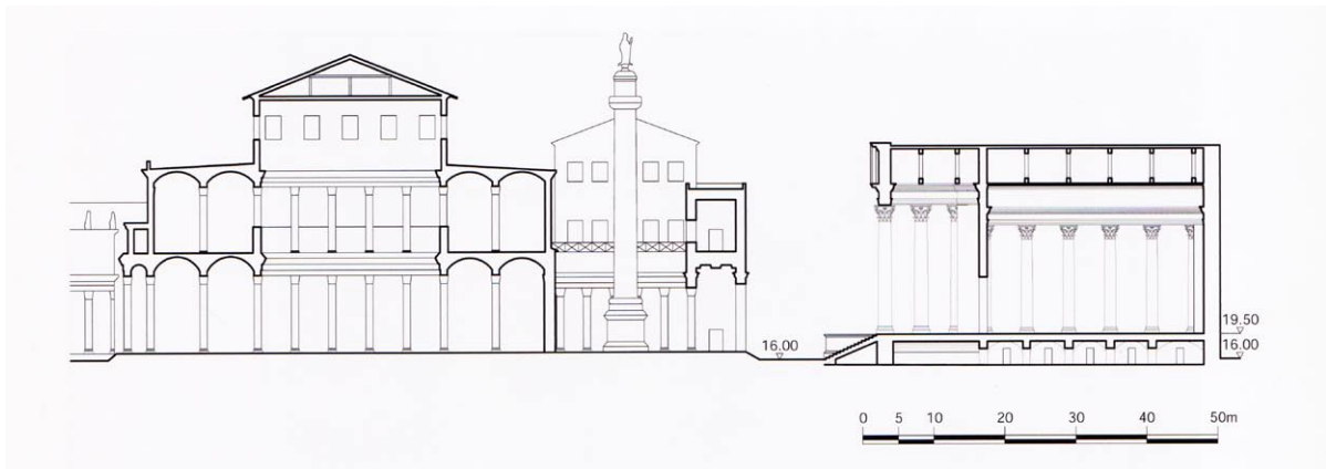
FIG. 10. Sezione longitudinale ricostruttiva del foro di Traiano e del templum divi Traiani, secondo la proposta di Paola Baldassarri (da Baldassarri 2016).
