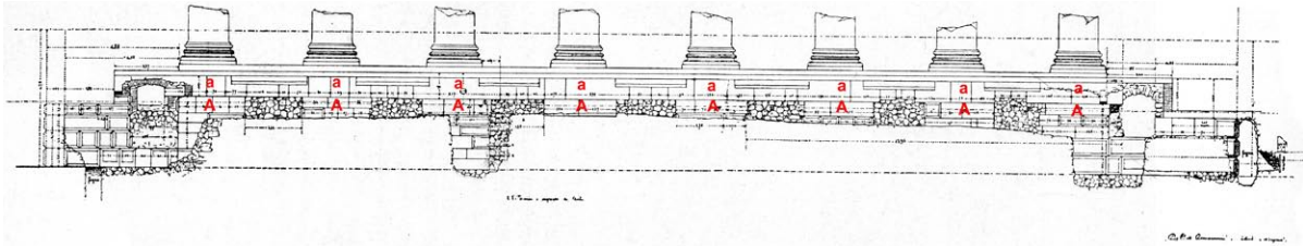
FIG. 15. Sezione trasversale della facciata del Pantheon (disegno di Pier Olindo Armanini). Sono segnalati con la A maiuscola le assise di fondazione in travertino del tempio augusteo; con la a minuscola la sopraelevazione delle assise di fondazione del tempio adrianeo (da La Rocca 2015).
