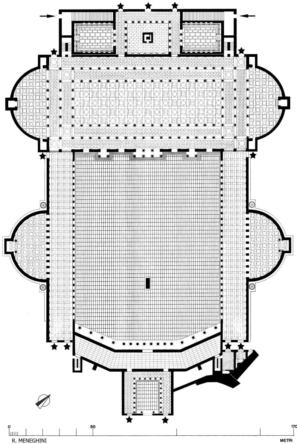
FIG. 27. Planimetria ricostruttiva del foro di Traiano. Con le stelle sono segnalati gli ingressi —alcuni dei quali ipotetici— al complesso forense (rilievo R. Meneghini).
