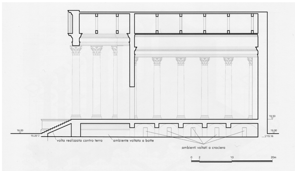
FIG. 18. Sezione longitudinale ricostruttiva del templum divi Traiani, secondo Paola Baldassarri (da Baldassarri 2016).
