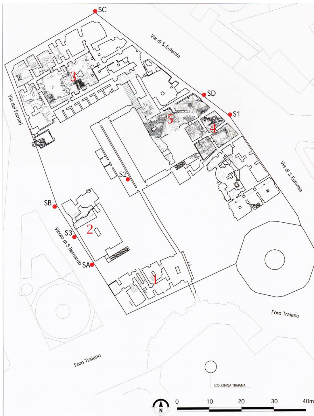
FIG. 17. Pianta del palazzo Valentini. 1: area delle ex-carceri; 2: area della ex-mensa; 3: area delle Piccole Terme C; 4: area della domus romana A; 5: area della domus romana B. Con i puntini sono segnalati i carotaggi compiuti intorno al palazzo e nel cortile.
