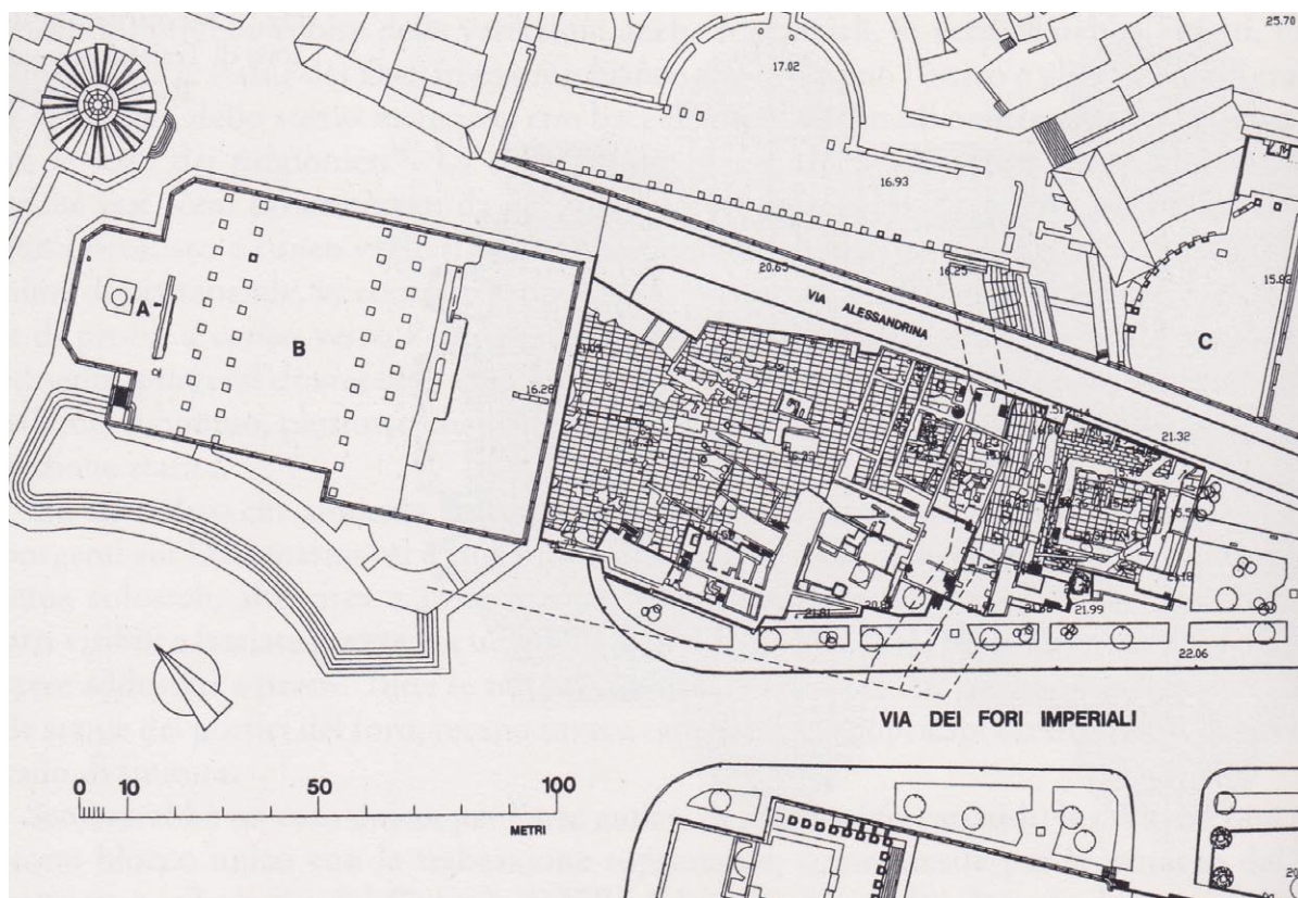
FIG. 25. Pianta dell'area archeologica del foro di Traiano. A sud, a linee tratteggiate, l'ubicazione della parete e della galleria trisegmentata. In alcuni tratti è visibile il letto di preparazione per l'applicazione di lastre pavimentali di marmo (rilievo R. Meneghini).
