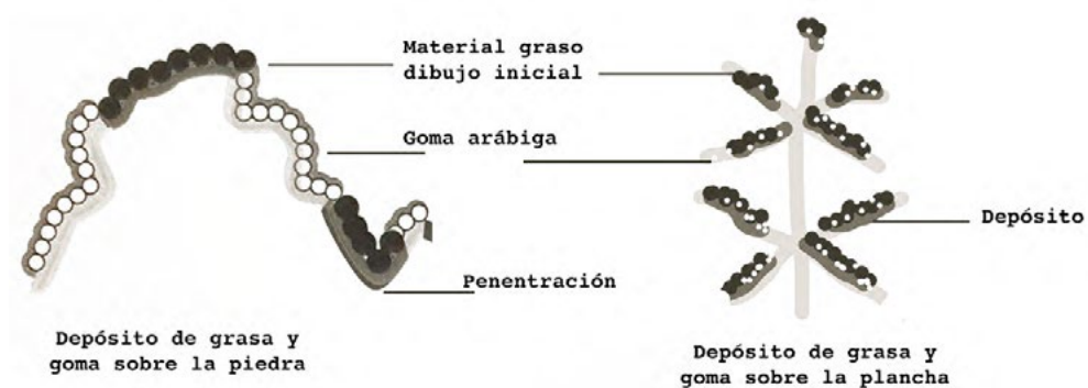
Figura 6. Gráfico comparativo de los depósitos del material graso sobre el grano de la piedra y sobre el grano del acero. Fuente: Imagen de la autora.
