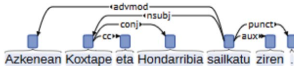
11. irudia. Azkenean Koxtape eta Hondarribia sailkatu ziren. esaldiaren dependentzia-zuhaitza DUetara egokitu ondoren.
