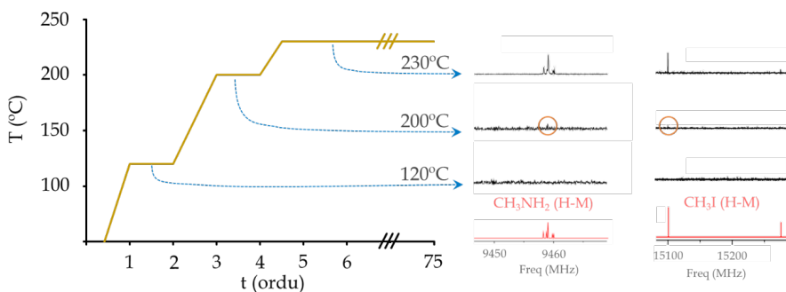
5. irudia. Tenperatura desberdinetan eta denbora-tarte desberdinetan lortutako \text{CH}_3\text{NH}_2 eta \text{CH}_3\text{I} molekulen espektro errotazionalaren zatia.
