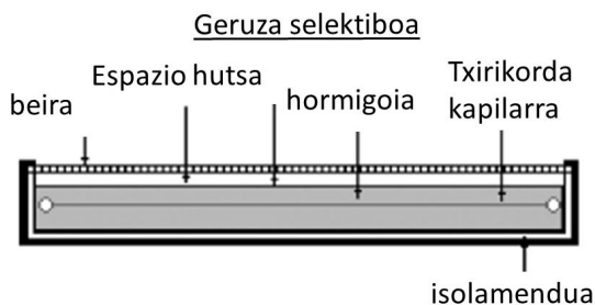
27. irudia. Biltegitatzeko eguzki-kolektorearen diagrama [35].
