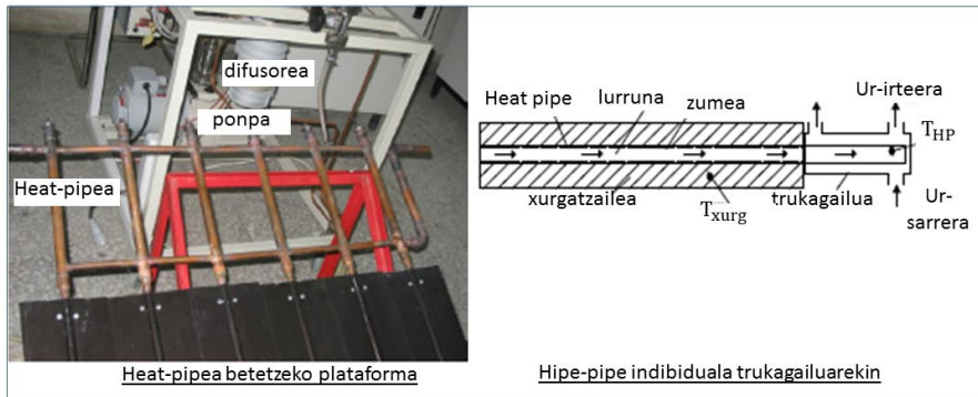
16. irudia. Bero-hodiaren konfigurazioa kobrezko hodian [21].
