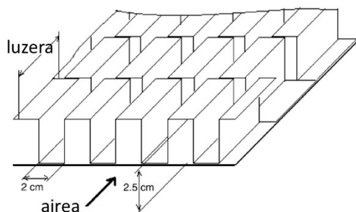
10. irudia. Xurgatzaileko hegalekin konfigurazioa [15].
