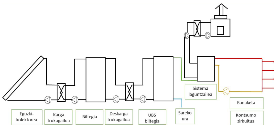
3. irudia. Eguzki-energia termikoaren eskema orokorra [8].
