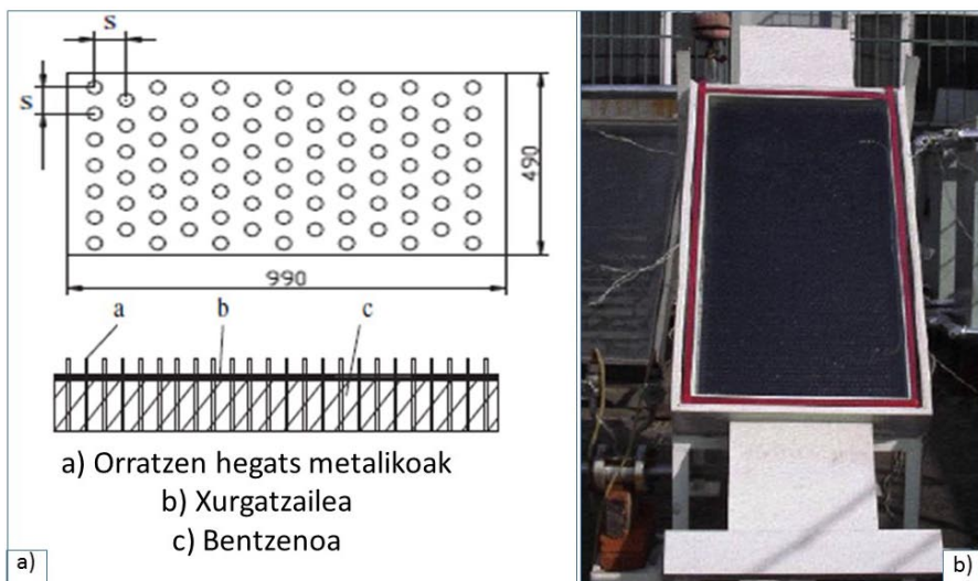
13. irudia. Orratzen hegaleko kolektoreak. a) Konfigurazioa eta b) Prototipoa [18]
