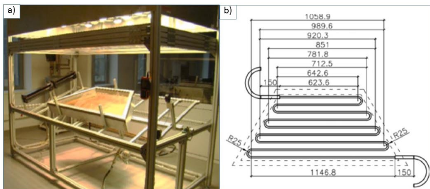
31. irudia. (a) Fatxada trapezoidala, eguzki-kolektoreekin integratua. (b) Meandro motako kobre jarraituaren konfigurazioa [39].
