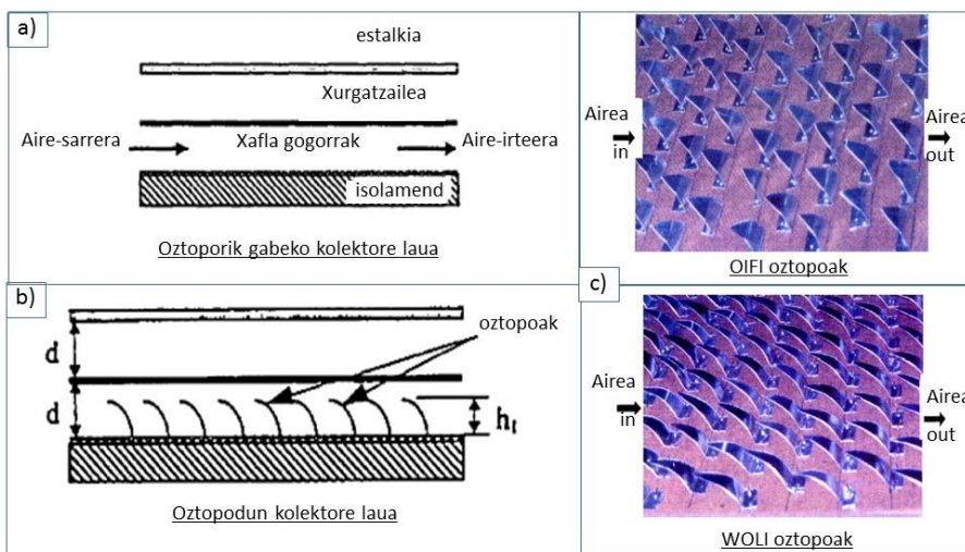
14. irudia. Kolektore lauaren konfigurazioa, (a) oztopoekin, (b) oztoporik gabe eta (c) oztopo batzuekin [19].
