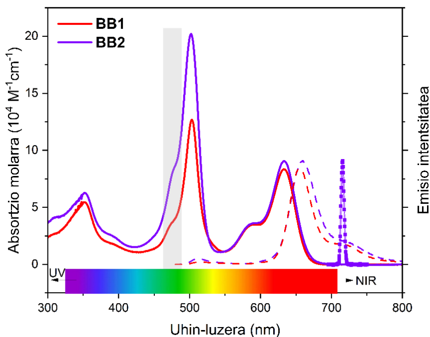
5. irudia. BB1 eta BB2 aren xurgapen- eta fluoreszentzia-espektoak (normalizatuak, kitzikapena emalearen eremuan, ikusi betegarri grisarekin nabarmendutako eremua) disoluzio diluituetan (dietyl eterrean, 2 \mu M ). Azken multikromoforoaren laser-espektoa ere (zirkuludun lerroa) irudikatu da.
